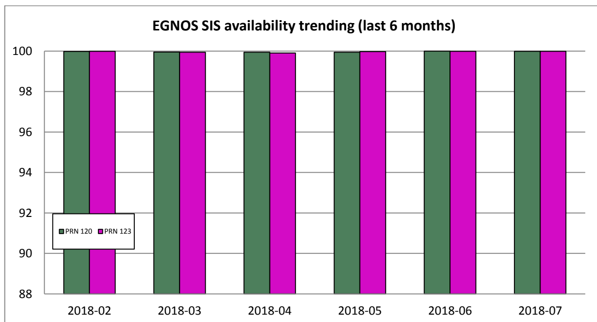
Figure 2 – Trend of EGNOS SIS Availability per GEO.
