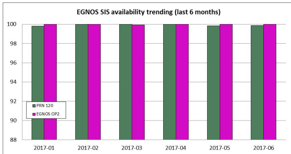
Figure 2 – Trend of EGNOS SIS Availability per GEO.
